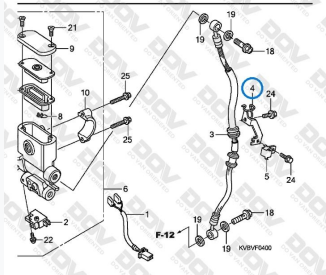
CYLINDER – XI LANH PHANH CHÍNH
