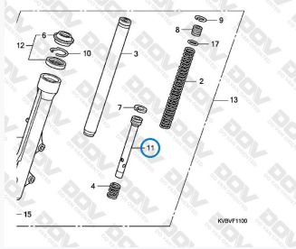
FRONT FORK- GIẢM XÓC TRƯỚC
